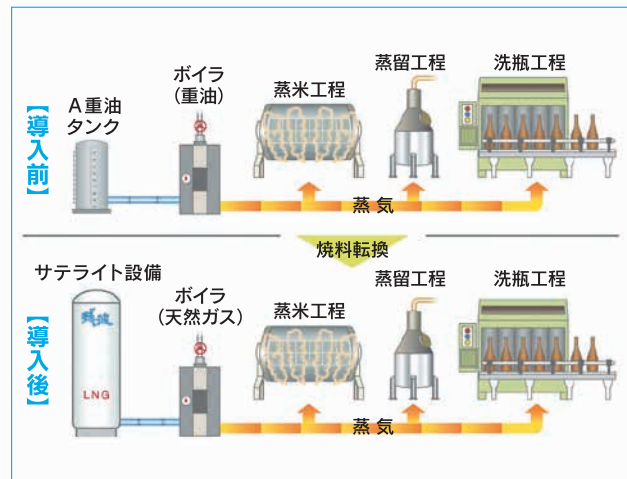
敷地奥に設置されたサテライト設備 最新の高效率ボイラに更新
